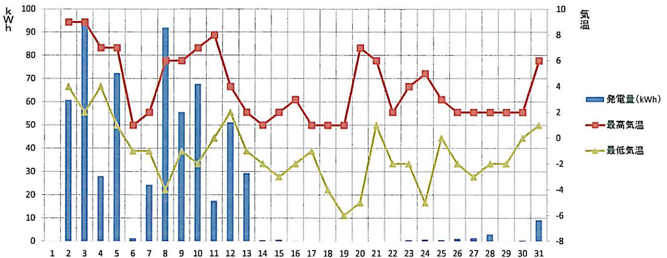
【2014年12月】須坂市消防本部 発電量と気温の推移
