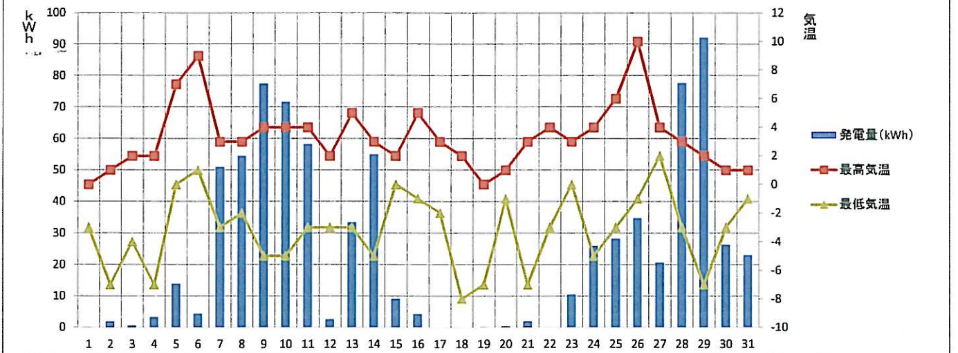
【2015年1月】須坂市消防本部 発電量と気温の推移
