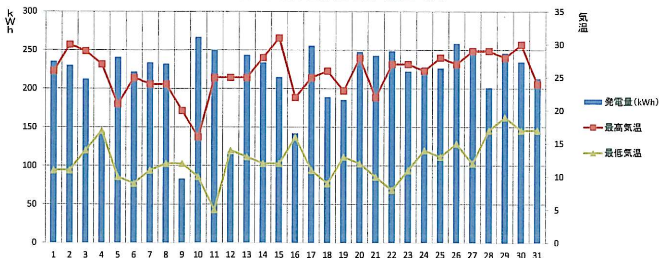
【2015年5月】須坂市消防本部 発電量と気温の推移
