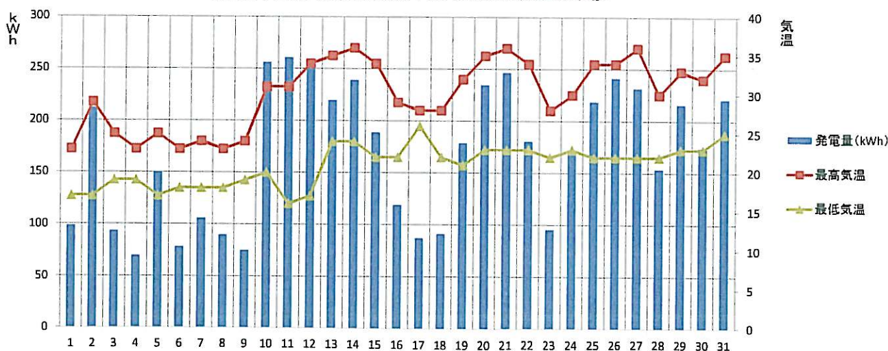
【2015年7月】須坂市消防本部 発電量と気温の推移
