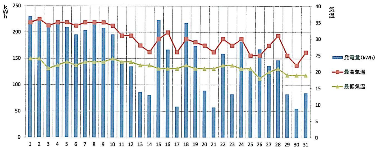
【2015年8月】須坂市消防本部 発電量と気温の推移
