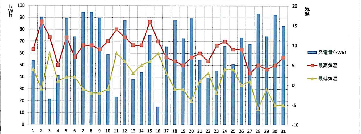
【2015年12月】須坂市消防本部 発電量と気温の推移
