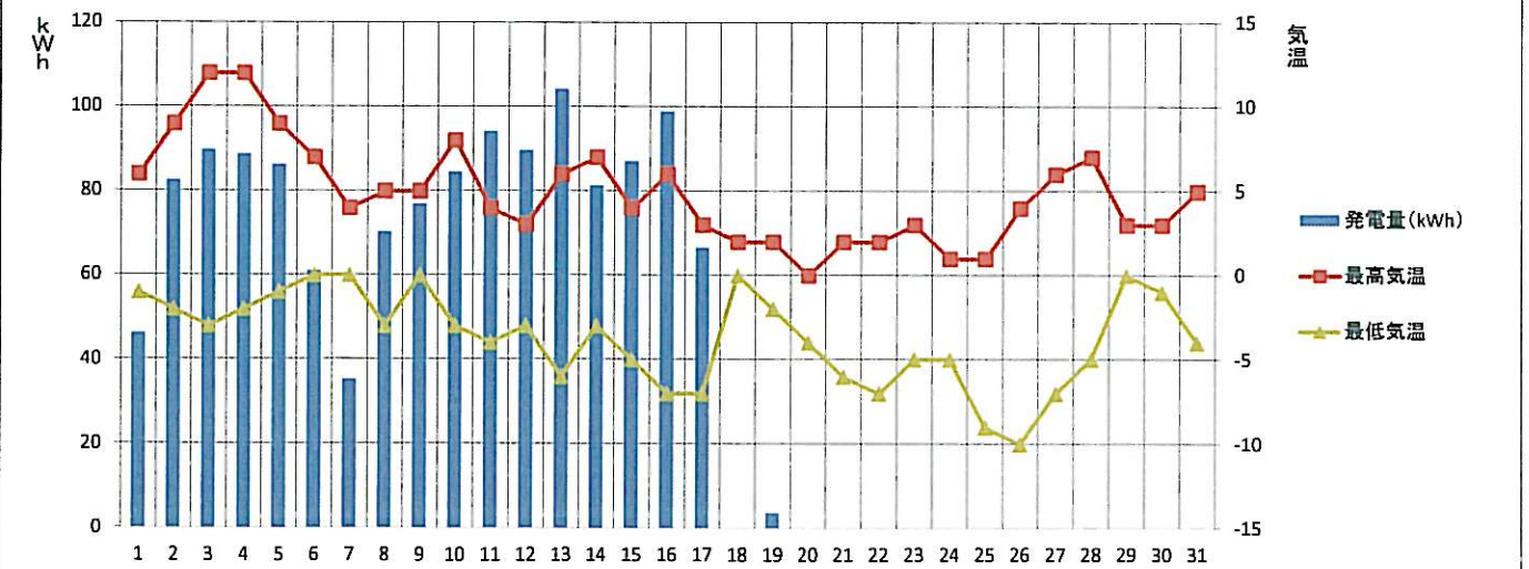
【2016年1月】須坂市消防本部 発電量と気温の推移
