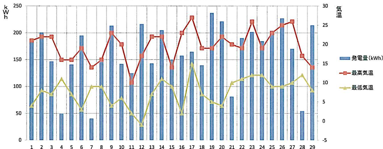
【2016年4月】須坂市消防本部 発電量と気温の推移
