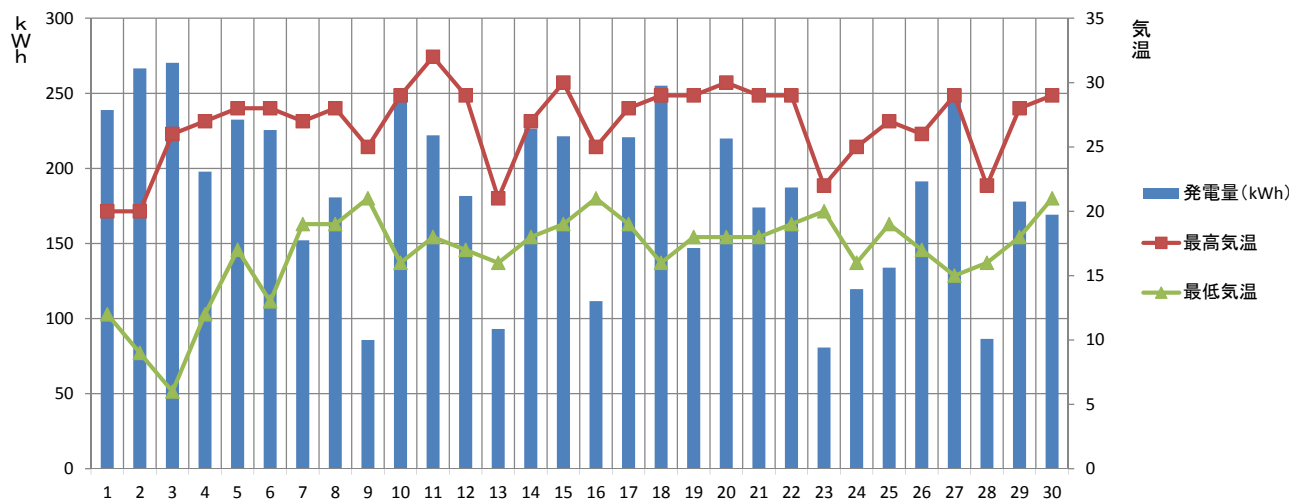
【2016年6月】須坂市消防本部 発電量と気温の推移
