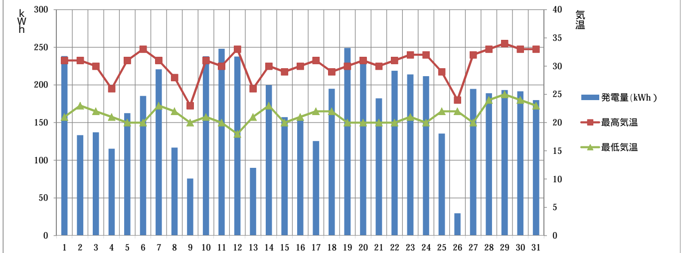
【2016年7月】須坂市消防本部 発電量と気温の推移
