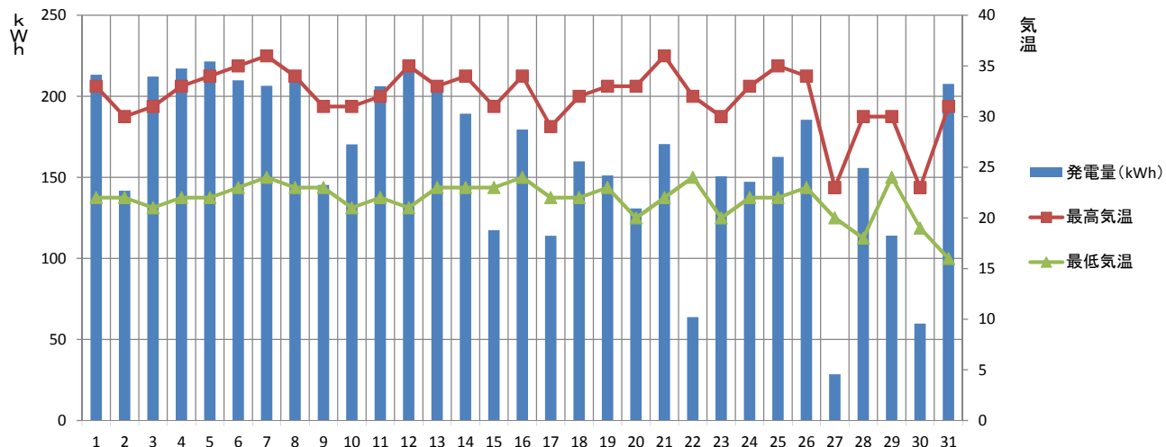
【2016年8月】須坂市消防本部 発電量と気温の推移
