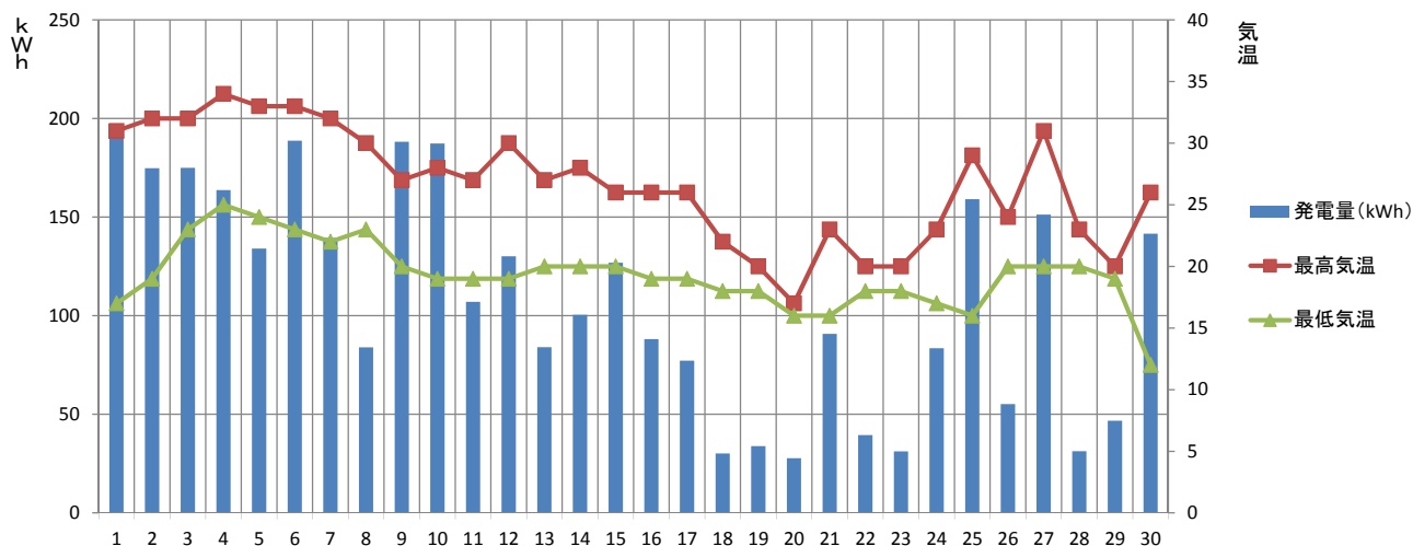
【2016年9月】須坂市消防本部 発電量と気温の推移
