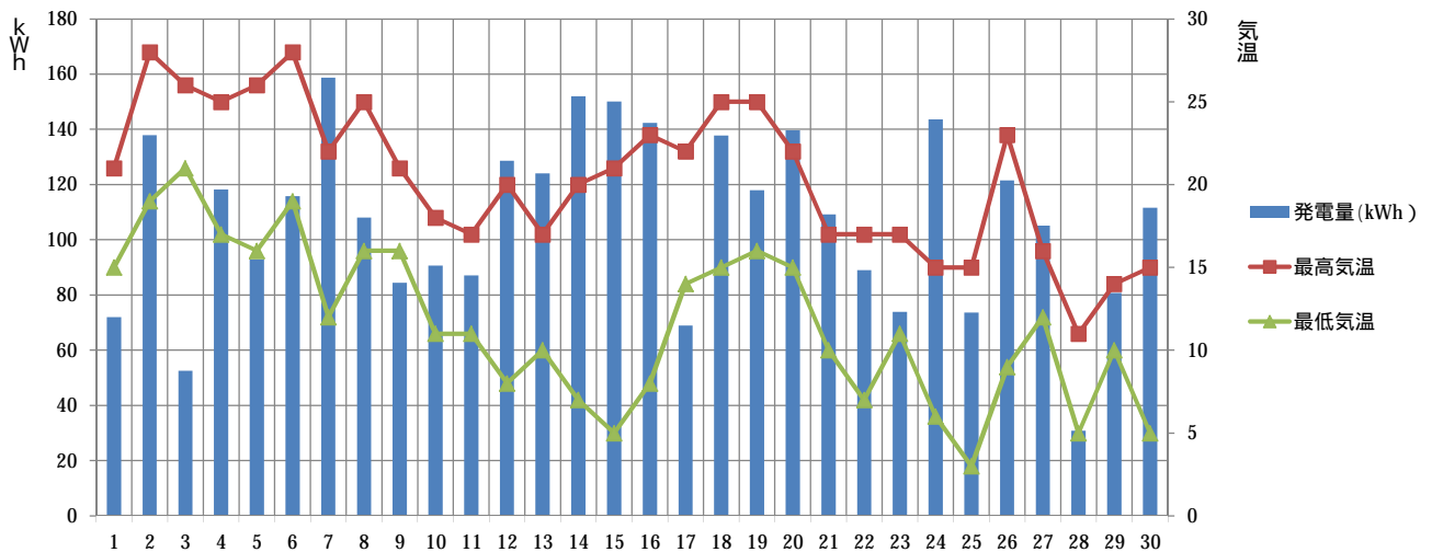
【2016年10月】須坂市消防本部 発電量と気温の推移
