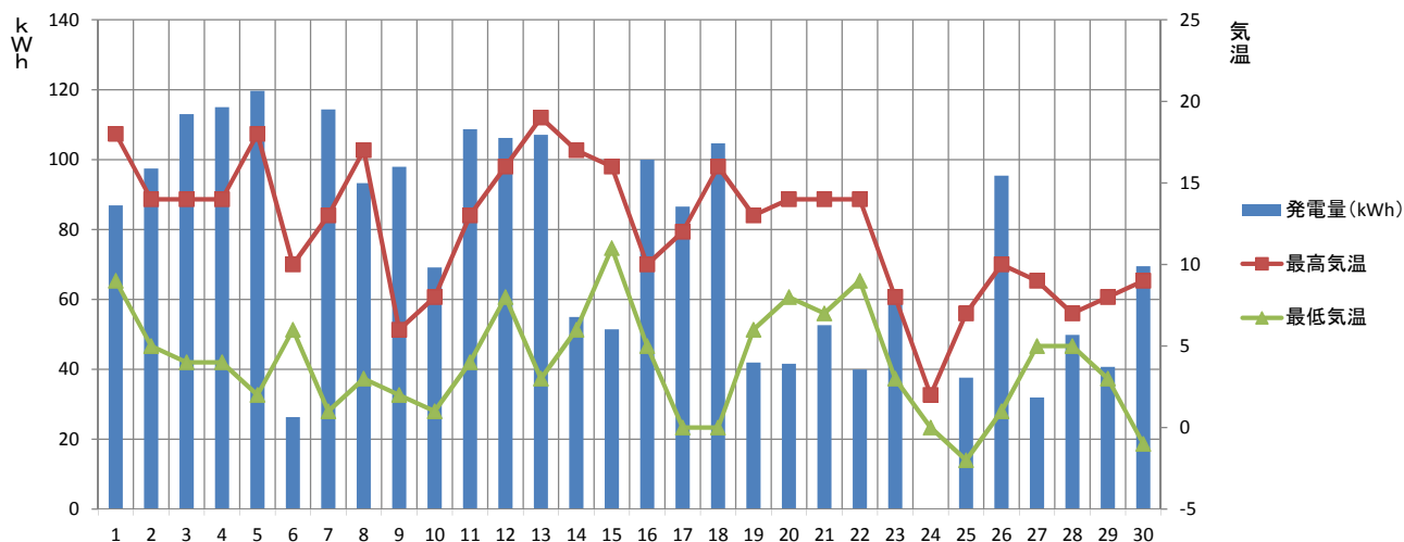
【2016年11月】須坂市消防本部 発電量と気温の推移
