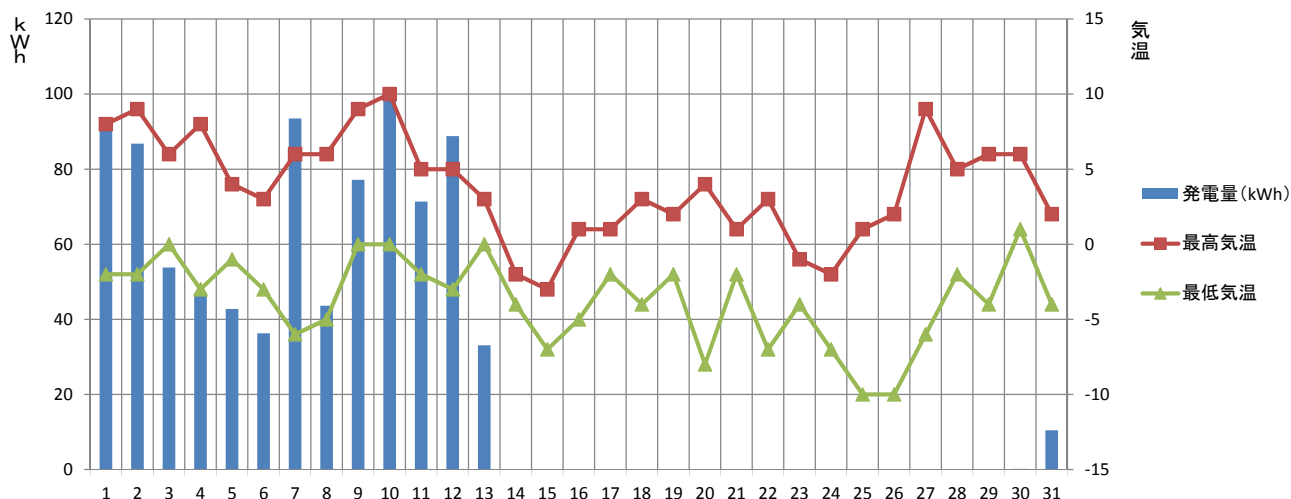
【2017年1月】須坂市消防本部 発電量と気温の推移
