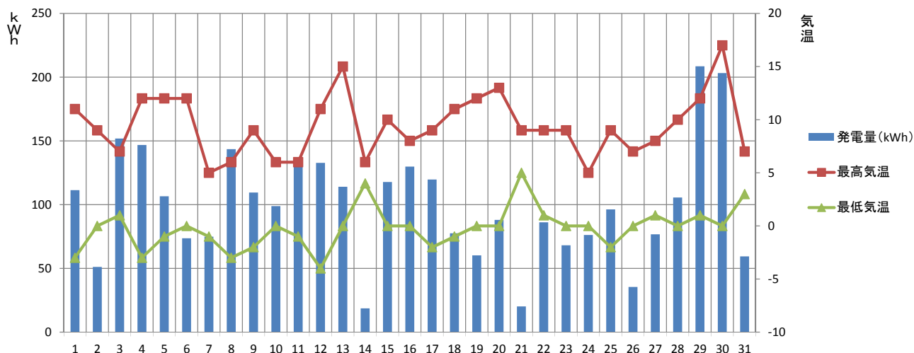
【2017年3月】須坂市消防本部 発電量と気温の推移
