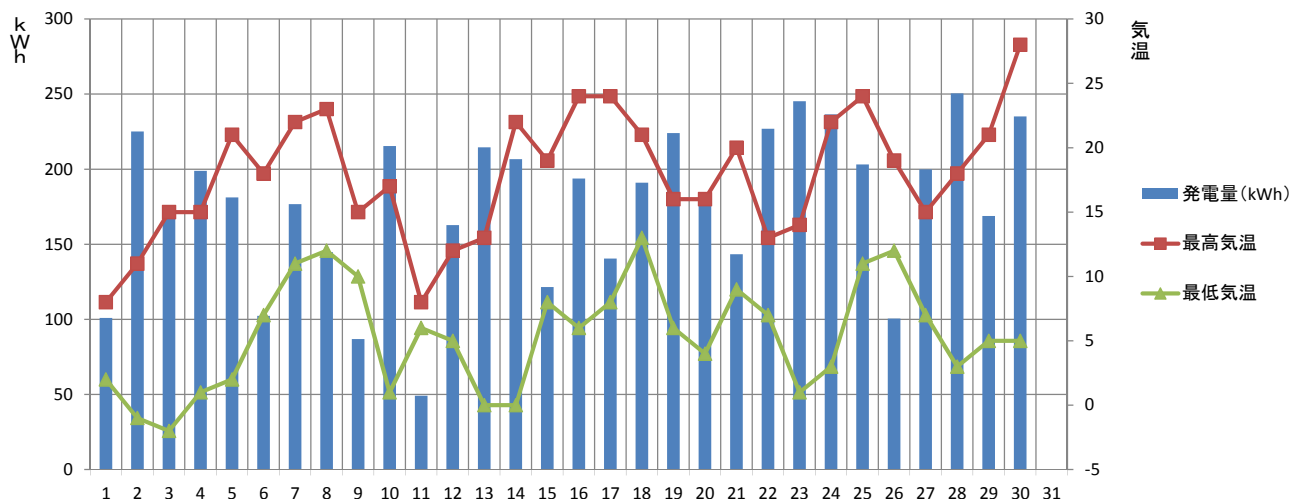
【2017年4月】須坂市消防本部 発電量と気温の推移
