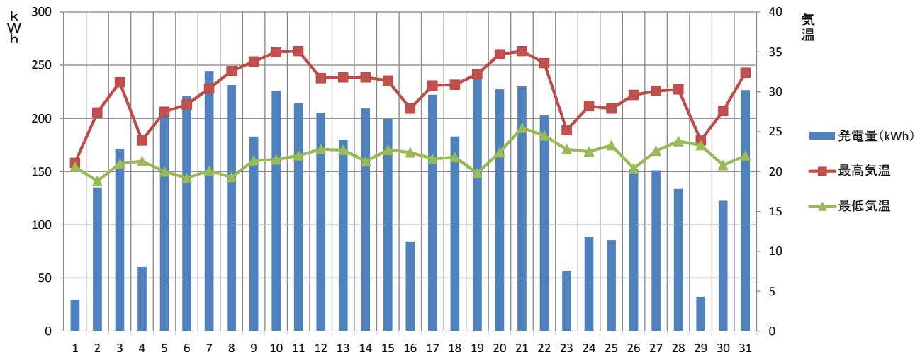
【2017年7月】須坂市消防本部 発電量と気温の推移
