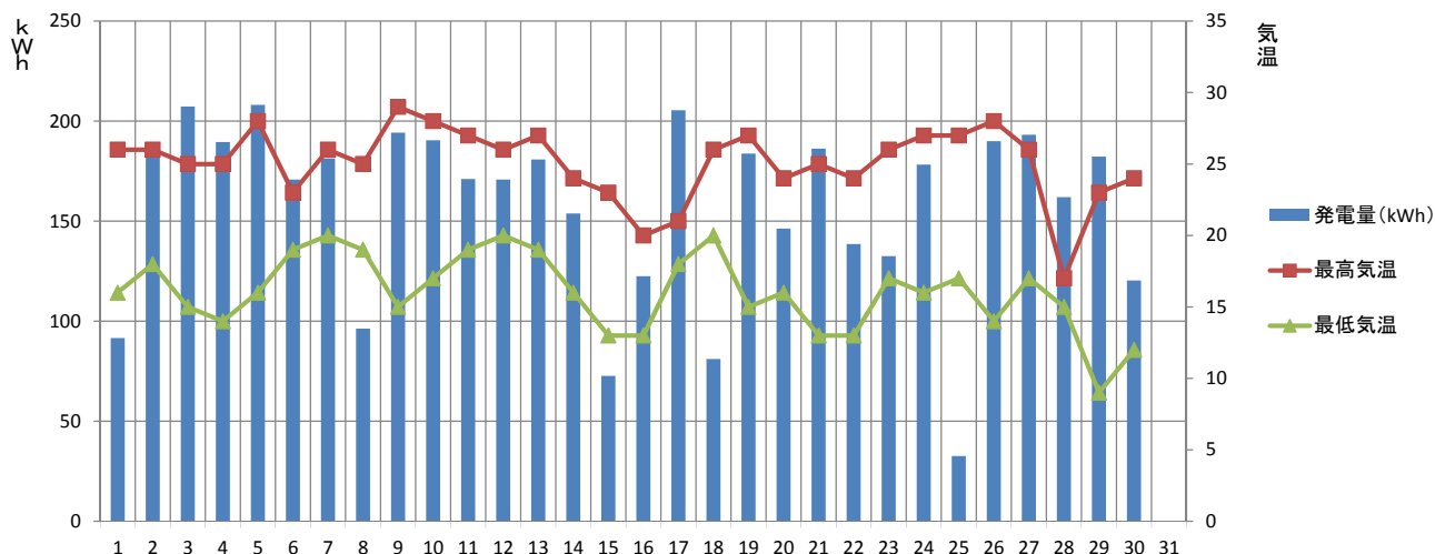
【2017年9月】須坂市消防本部 発電量と気温の推移
