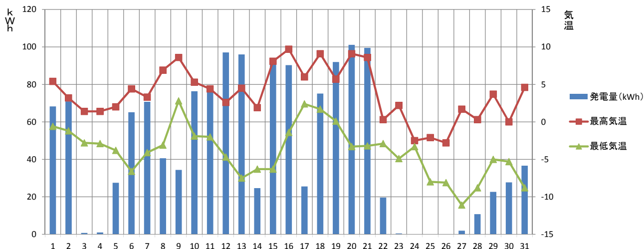
【2018年1月】須坂市消防本部 発電量と気温の推移
