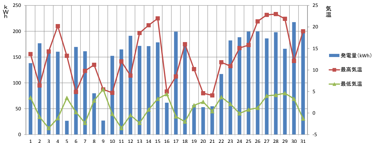
【2018年3月】須坂市消防本部 発電量と気温の推移
