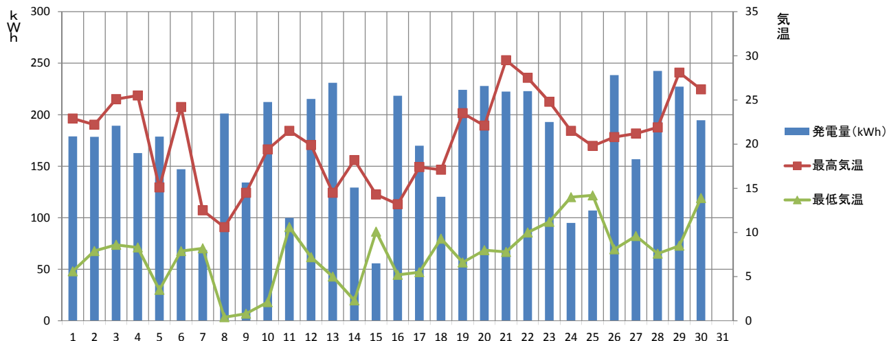
【2018年4月】須坂市消防本部 発電量と気温の推移
