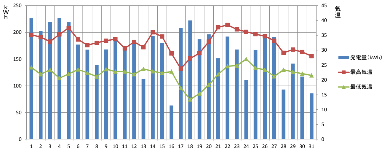
【2018年8月】須坂市消防本部 発電量と気温の推移
