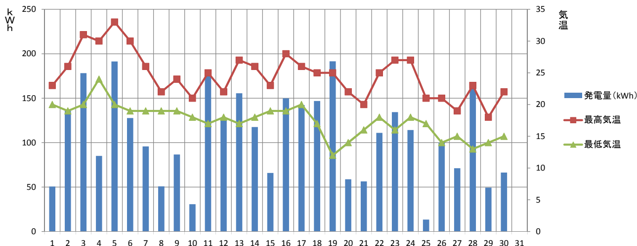
【2018年9月】須坂市消防本部 発電量と気温の推移
