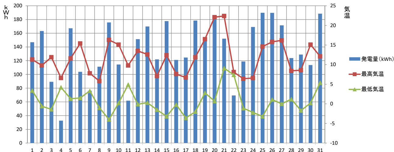
【2019年2月】須坂市消防本部 発電量と気温の推移
