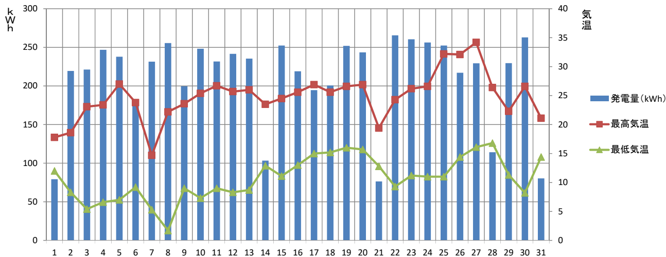
【2019年5月】須坂市消防本部 発電量と気温の推移
