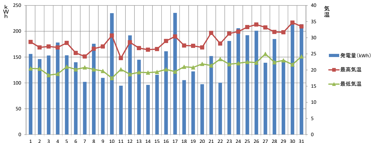
【2019年7月】 須坂市消防本部 発電量と気温の推移
