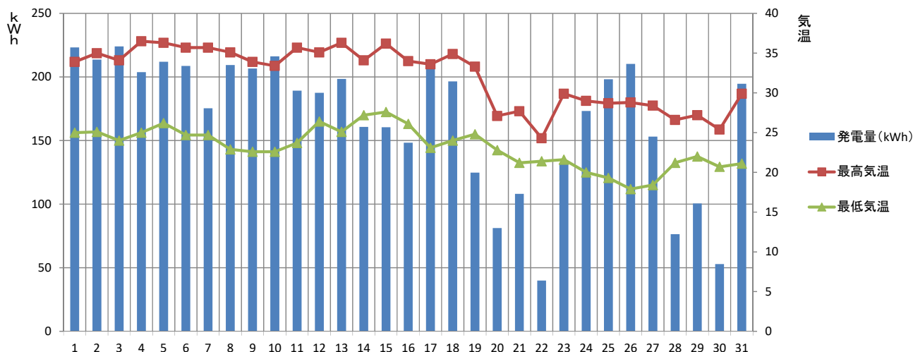
【2019年8月】須坂市消防本部 発電量と気温の推移
