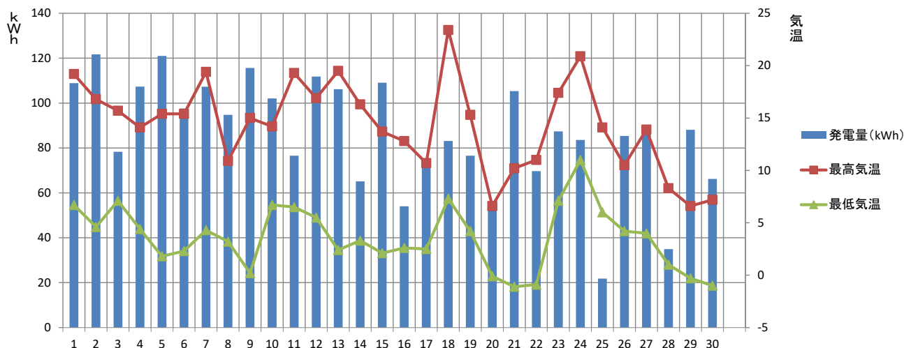
【2019年11月】須坂市消防本部 発電量と気温の推移
