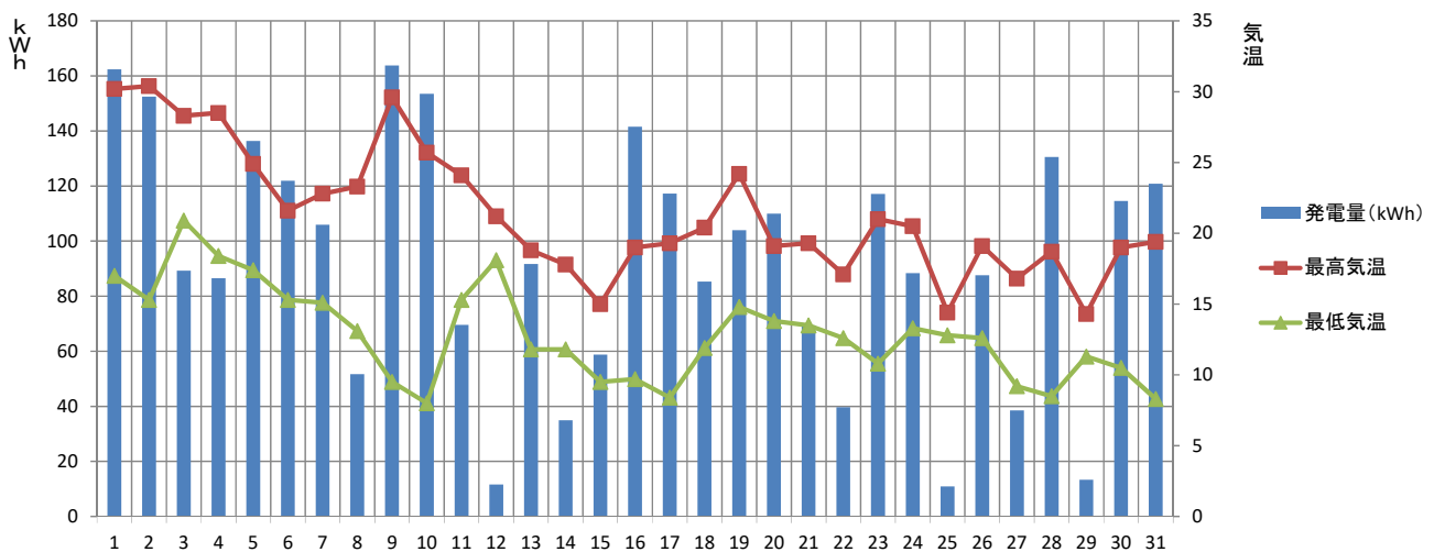
【2019年10月】須坂市消防本部 発電量と気温の推移
