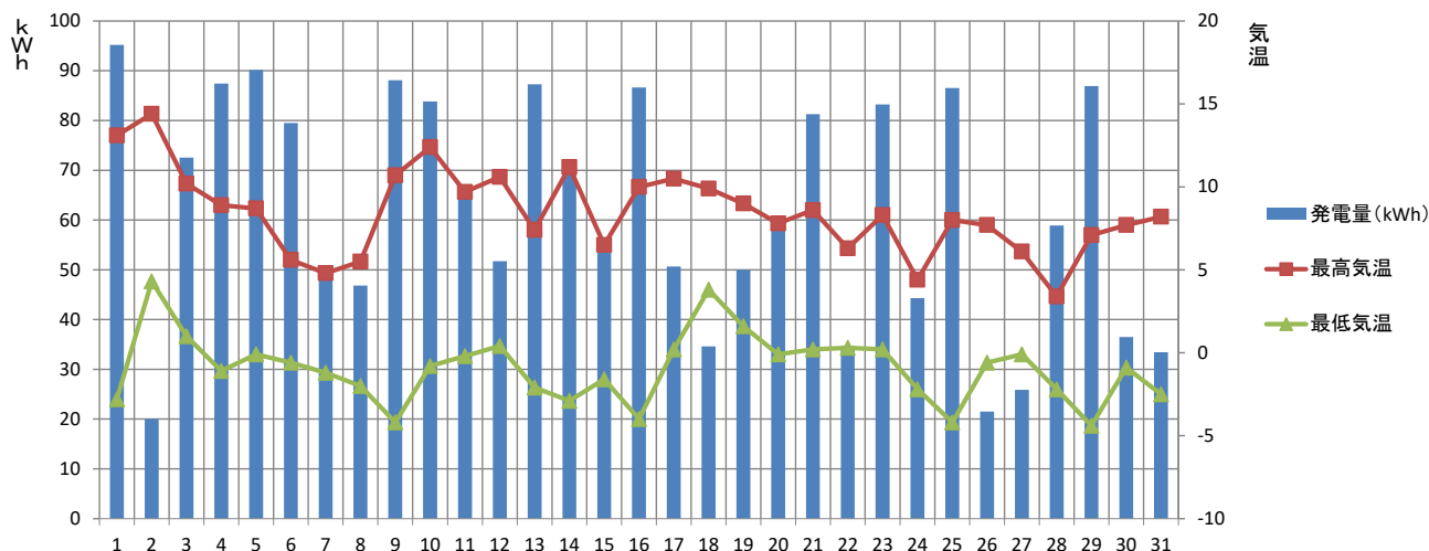
【2019年12月】須坂市消防本部 発電量と気温の推移
