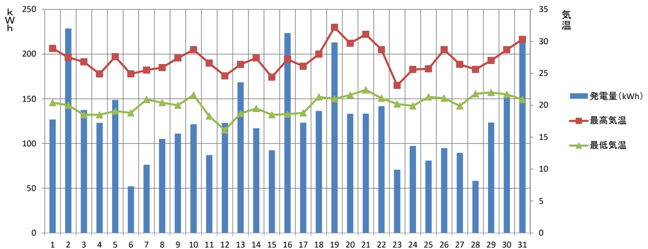
【2020年7月】須坂市消防本部 発電量と気温の推移
