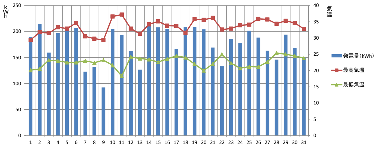
【2020年8月】須坂市消防本部 発電量と気温の推移
