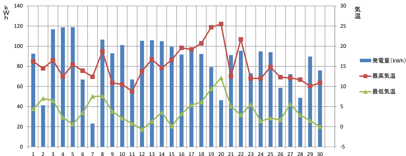
【2020年11月】 須坂市消防本部 発電量と気温の推移
