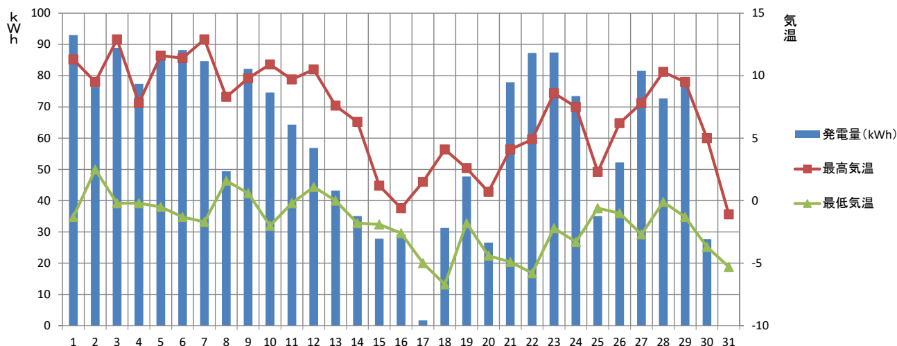
【2020年12月】須坂市消防本部 発電量と気温の推移
