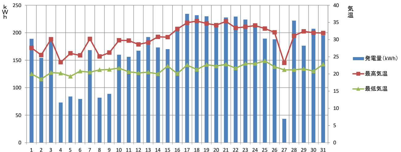
【2021年7月】須坂市消防本部 発電量と気温の推移
