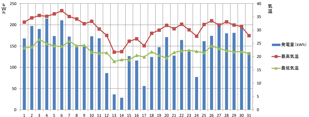
【2021年8月】須坂市消防本部 発電量と気温の推移
