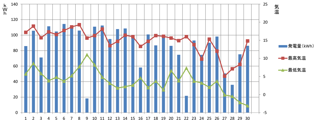
【2021年11月】須坂市消防本部 発電量と気温の推移
