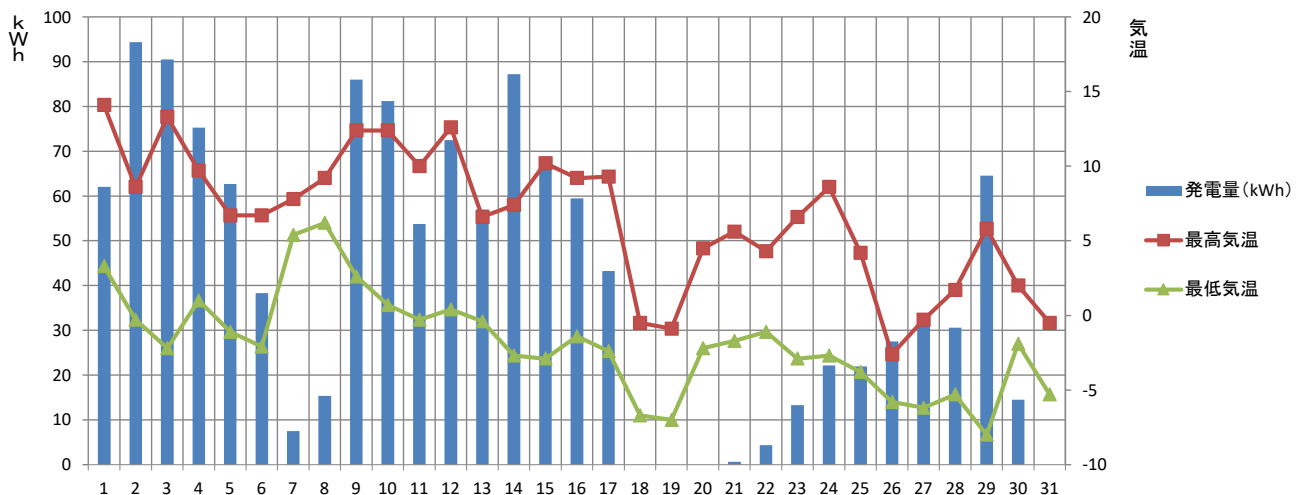
【2021年12月】須坂市消防本部 発電量と気温の推移
