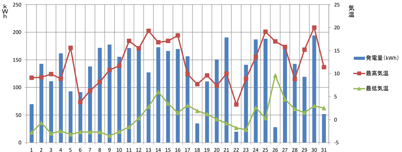
【2022年3月】須坂市消防本部 発電量と気温の推移
