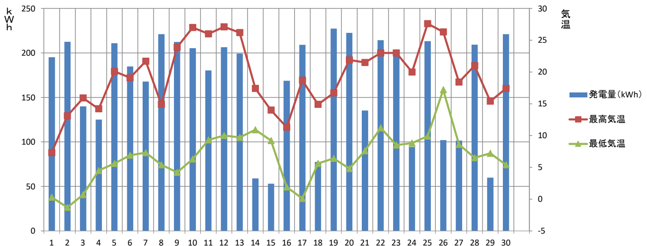
【2022年4月】須坂市消防本部 発電量と気温の推移
