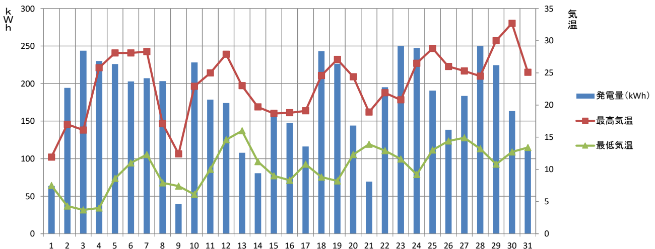
【2022年5月】須坂市消防本部 発電量と気温の推移
