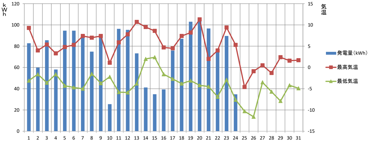
【2023年1月】 須坂市消防本部 発電量と気温の推移
