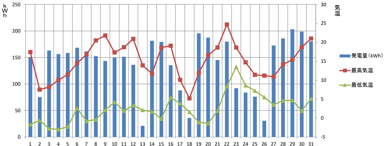
【2023年3月】 須坂市消防本部 発電量と気温の推移
