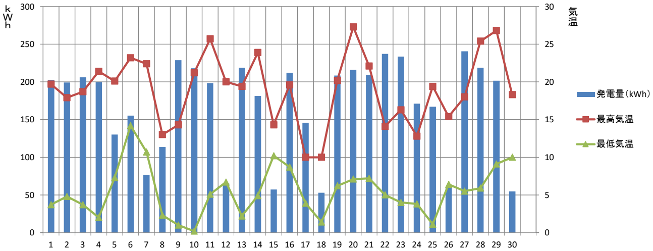
【2023年 4月】 須坂市消防本部 発電量と気温の推移
