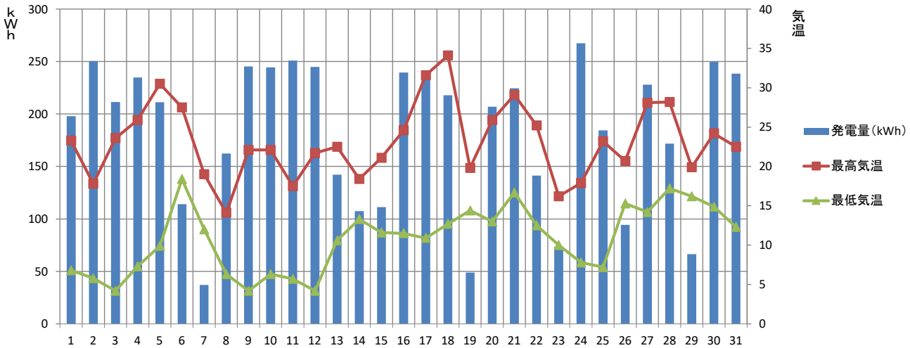
【2023年 5月】 須坂市消防本部 発電量と気温の推移
