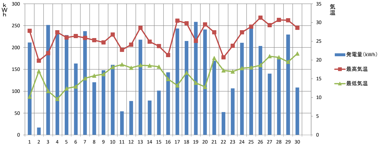
【2023年 6月】 須坂市消防本部 発電量と気温の推移
