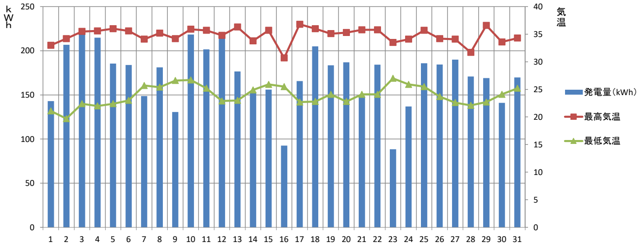
【2023年 8月】 須坂市消防本部 発電量と気温の推移
