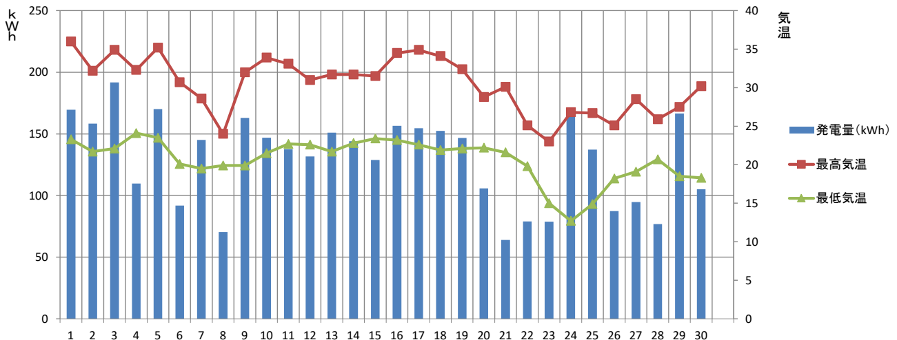
【2023年 9月】 須坂市消防本部 発電量と気温の推移
