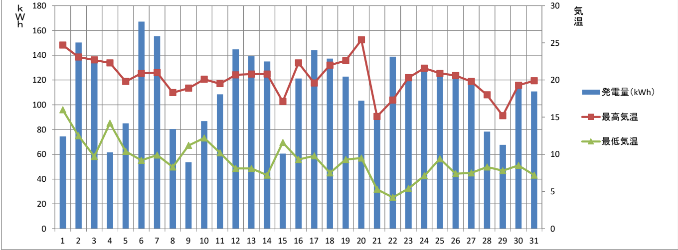
【2023年10月】 須坂市消防本部 発電量と気温の推移
